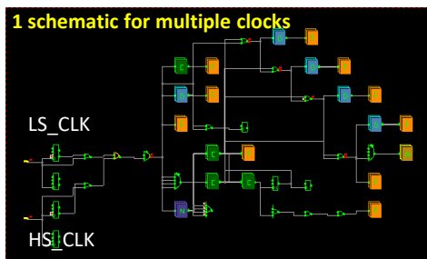
时钟组的 Schematic 展示
