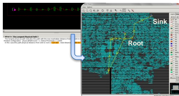
时钟综合质量分析: 定位最长时钟路径在物理版图的分布
