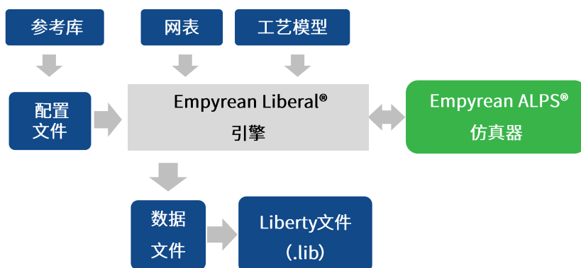
Empyrean Liberal®单元库特征化提取流程
